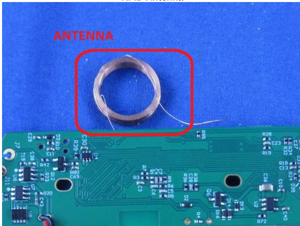
RFID Antenna
