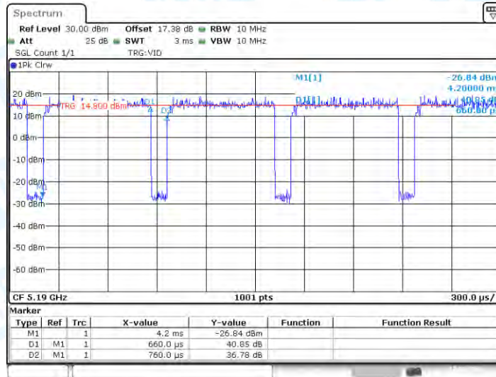
11AC40MIMO_Ant1_5190
