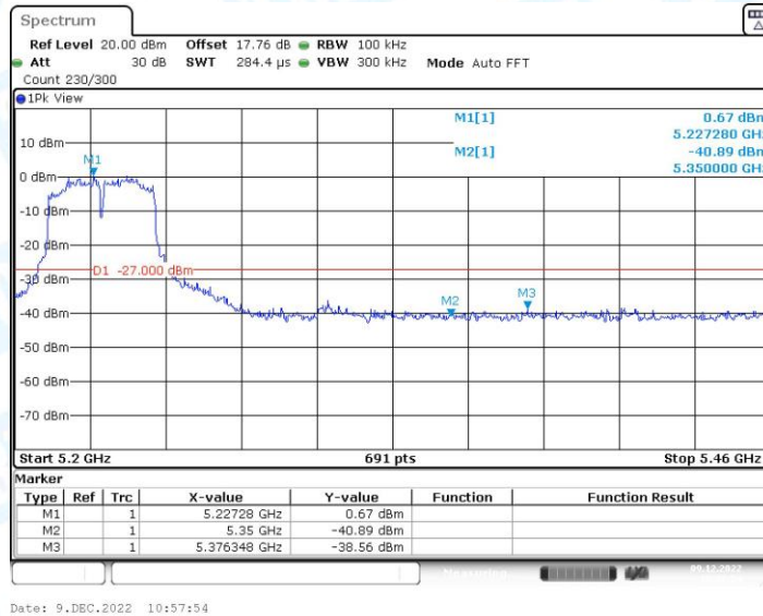
11AC80MIMO_Ant1_Low_5210
