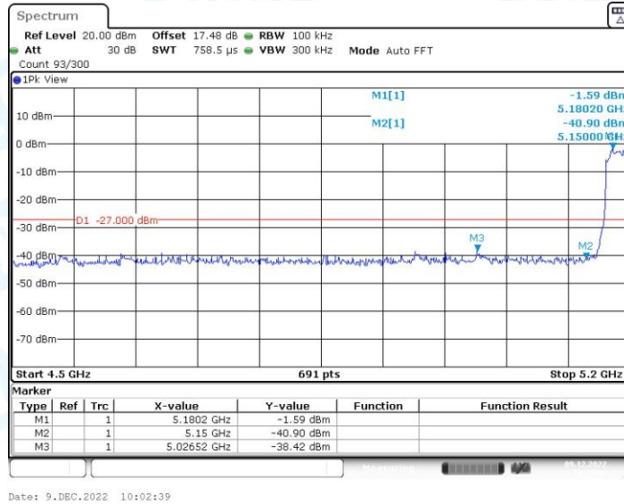
11N40MIMO_Ant2_Low_5190
