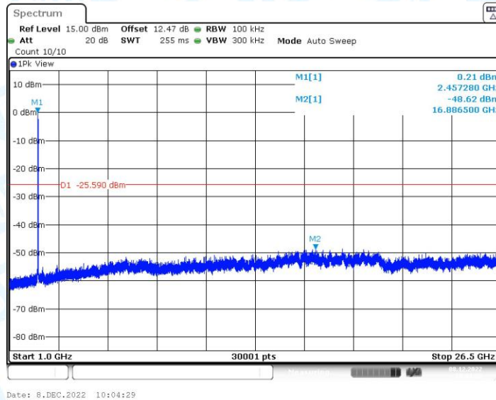
11N20MIMO_Ant2_2462_0~Reference
