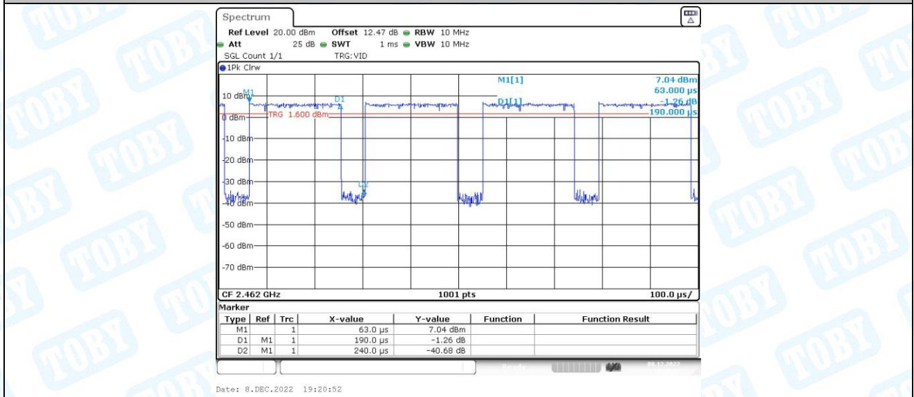
11G-CDD_Ant2_2462
