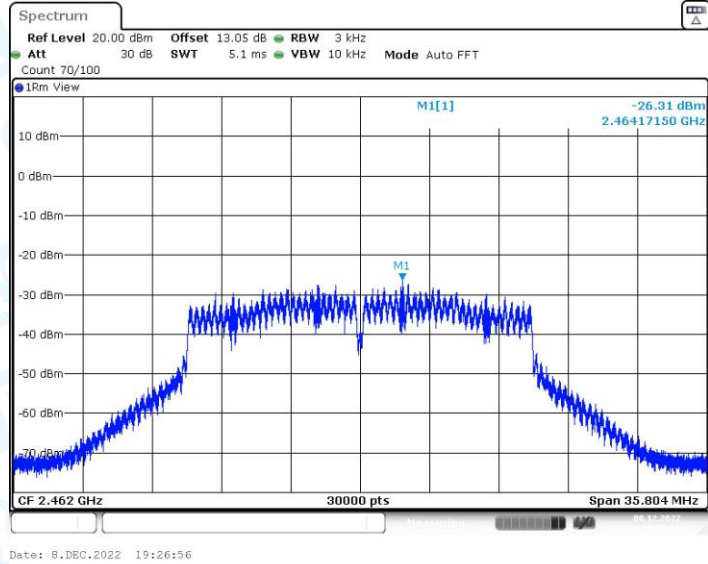
11N20MIMO_Ant2_2462
