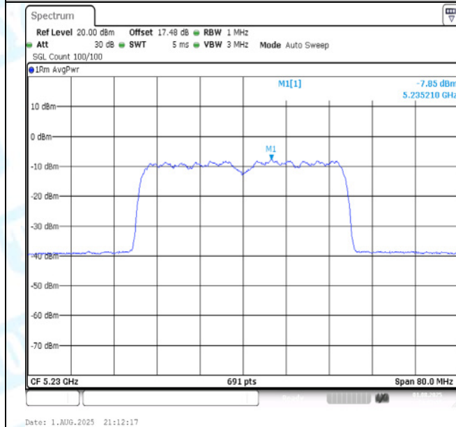
11AX40MIMO-Ant1-5230-PASS
