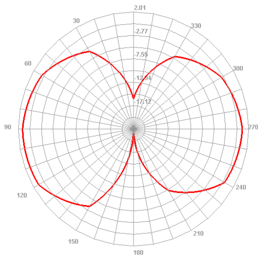
2450.000MHz E1
