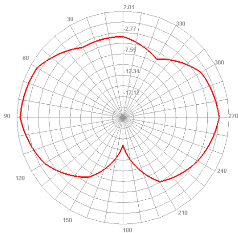
2450.000MHz E2
