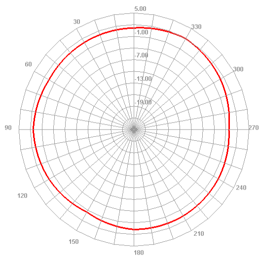
2450.000MHz H
