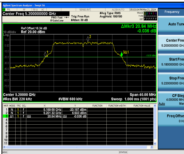
11A-Ant1-5200
