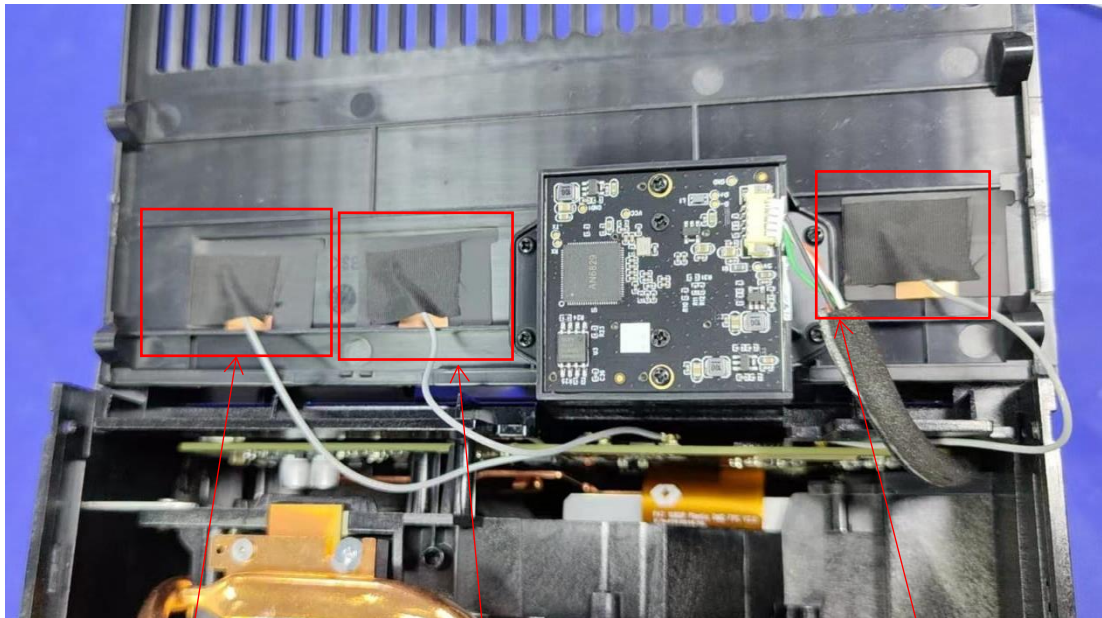
BT ANT
