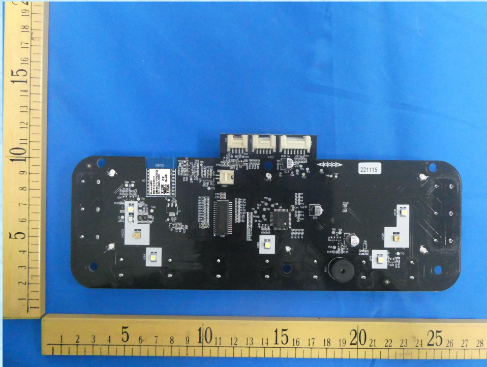
EUT Photo
