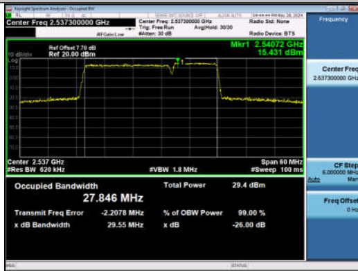
7-7-20MHz-10MHz-QPSK-QPSK-21051-21195-100RB#0- 50RB#0-PASS
