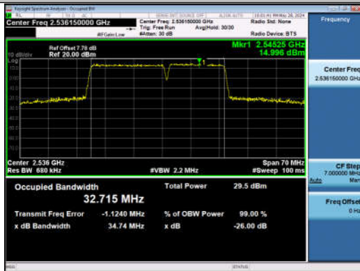
7-7-20MHz-15MHz-QPSK-QPSK-21026-21197-100RB#0- 75RB#0-PASS
