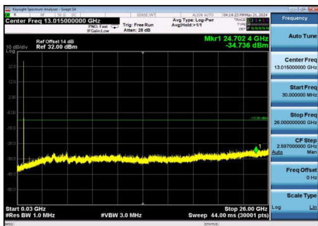
FDD17_HighRange_10MHz_30MHz~26GHz
