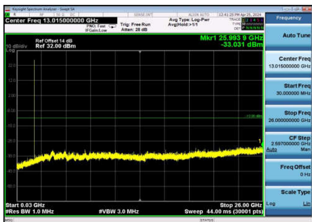
FDD25_HighRange_20MHz_30MHz~26GHz
