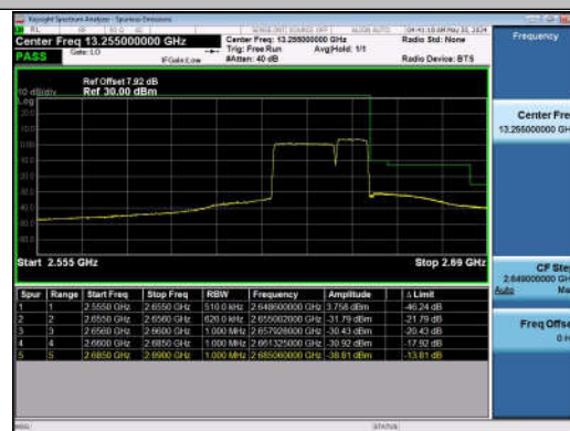
20MHz-10MHz_QPSK@QPSK-QPSK@QPSK_41041-41185 _100RB#0@100RB#0-50RB#0@50RB#0
