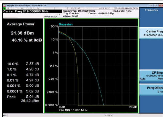
FDD26_Part 90_MidRange_10MHz_819_OneRB_high_Q16
