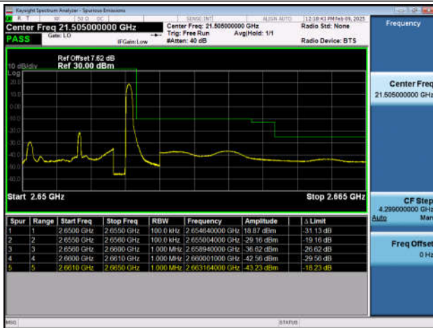
Band41_10MHz_QPSK_40290_1RB#0
