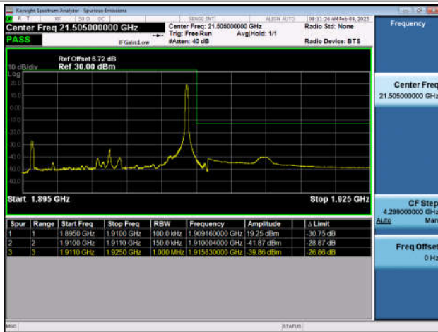
Band2_20MHz_QPSK_18700_1RB#0
