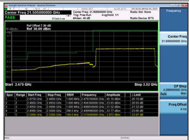
Band7_20MHz_QPSK_20850_100RB#0
