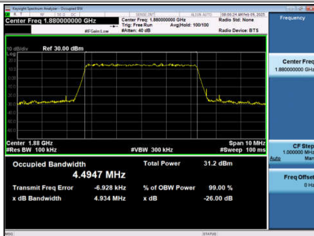
Band2-5MHz-QPSK-18900-25RB#0-PASS
