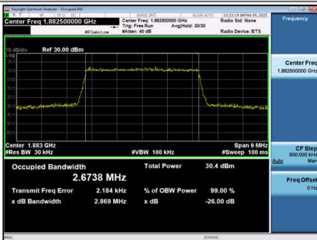
Band25-3MHz-QPSK-26365-15RB#0-PASS
