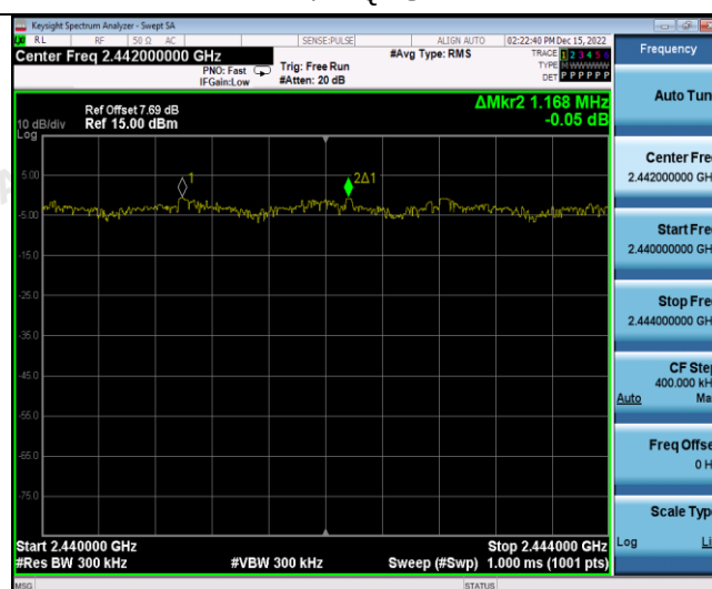
8DPSK
