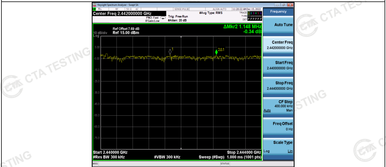
\pi/4 DQPSK
