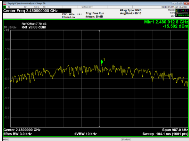
1Mbps / 2480MHz
