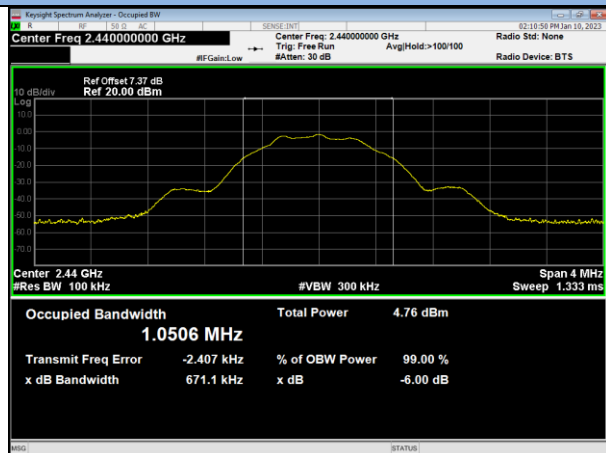
1Mbps / 2440MHz
