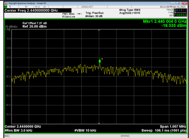
1Mbps / 2440MHz
