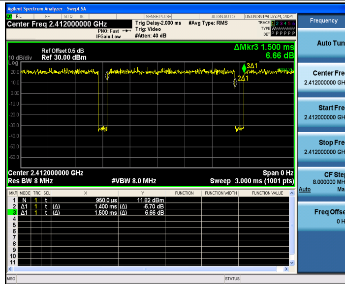
802.11g_Ant2_2412
