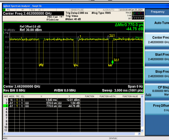
802.11n(HT20)_Ant2_2462
