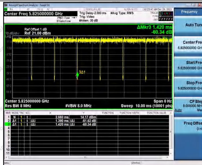
11A_Ant3_5825
