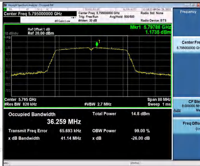
11AC40SISO_Ant2_5795
