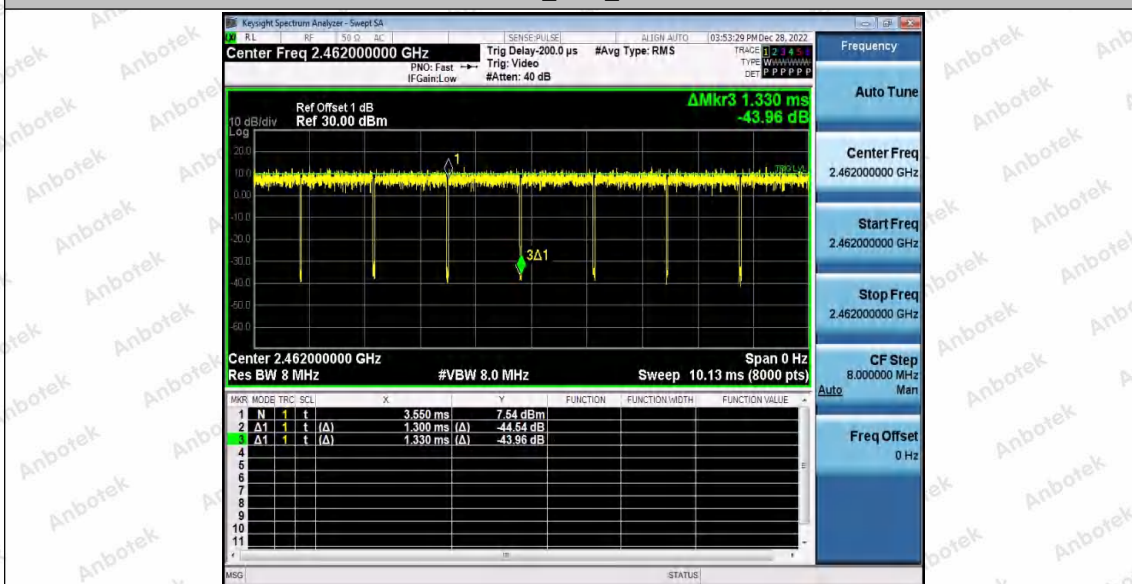
11N20_Ant3_2462
