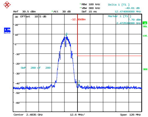
b_2472MHz_Chain 1 49.01dB
