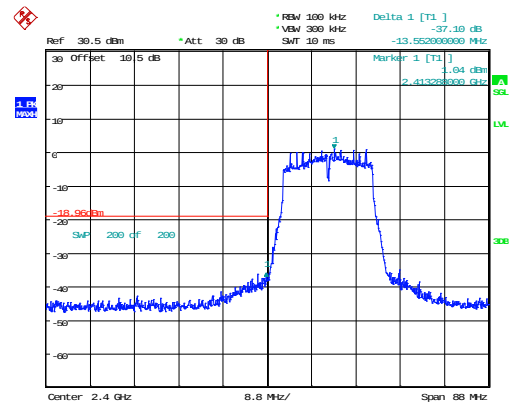
n20_2412MHz_Chain 1 37.10dB
