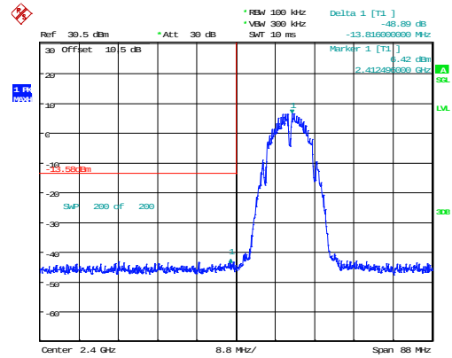
b_2412MHz_Chain 1 48.89dB
