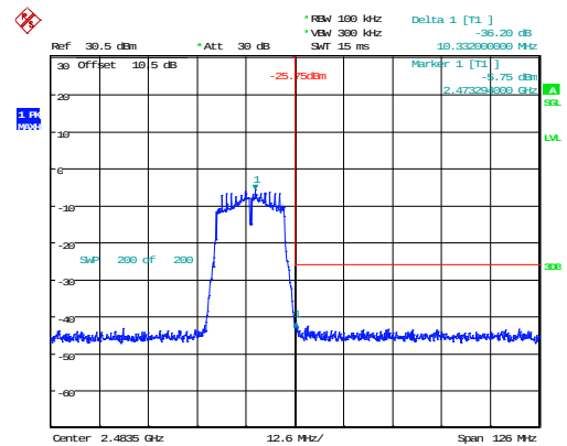
n20_2472MHz_Chain 1 36.20dB
