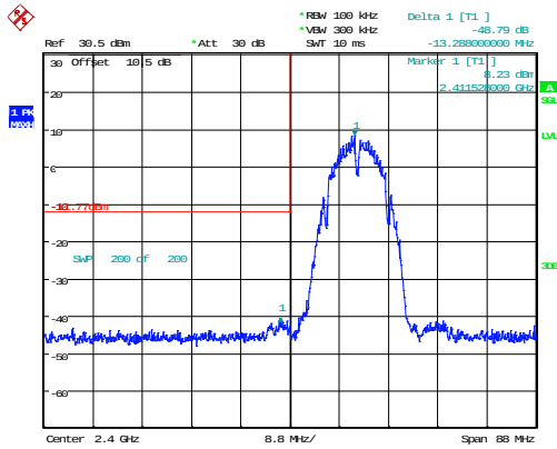
b_2412MHz_Chain 0 48.79dB
