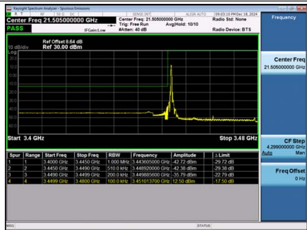
NTNV-n77(3450-3550)-PC3-30-30-L-DFT-BPSK-Edge_1RB_L eft-PASS
