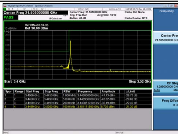
NTNV-n78(3450-3550)-PC2-30-70-L-DFT-BPSK-Edge_1RB_L eft-PASS
