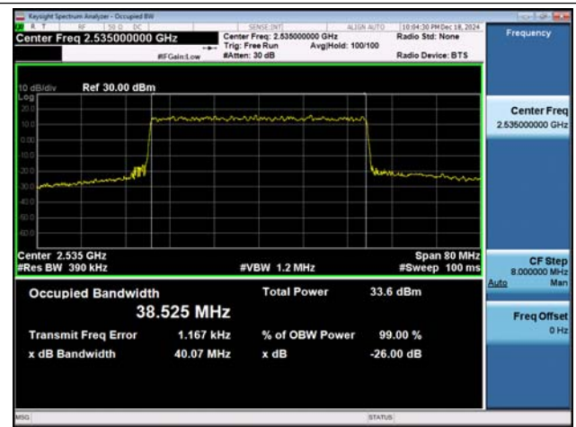
NTNV-n7-PC3-15-40-M-DFT-QPSK-Outet1-PASS
