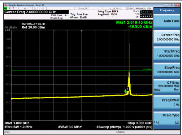
Band41_20MHz_QPSK_41490_1RB#0_1000~3000_1000~3 000
