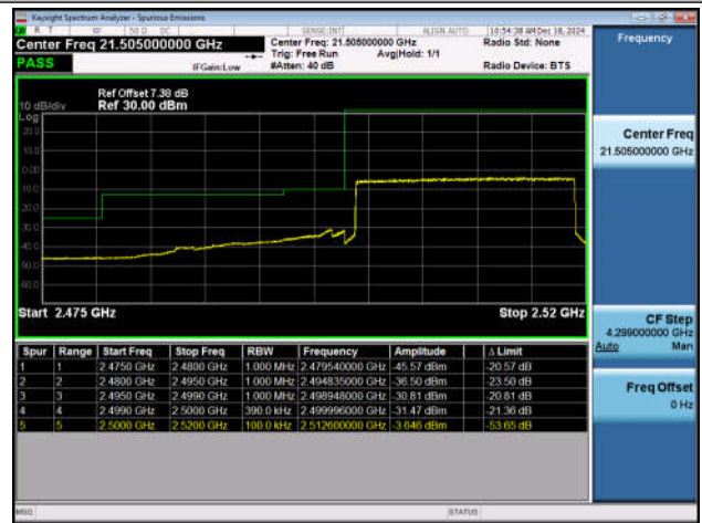
Band7_20MHz_QPSK_21350_100RB#0
