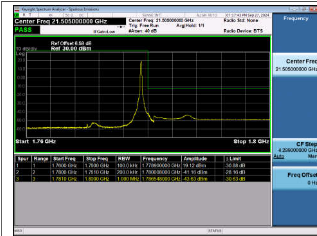
Band66_20MHz_QPSK_132572_1RB#99
