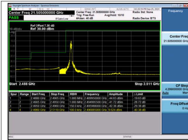
Band41_15MHz_QPSK_39725_1RB#0
