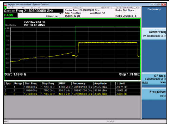
Band66_20MHz_QPSK_132072_100RB#0
