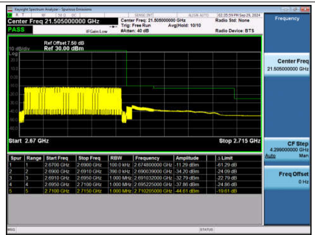
Band41_20MHz_QPSK_41490_100RB#0
