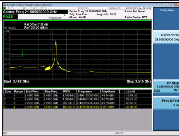
Band41_20MHz_QPSK_39750_1RB#0
