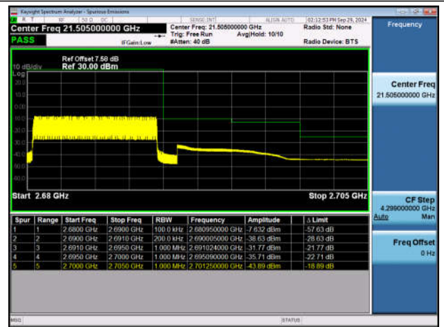
Band41_10MHz_QPSK_41540_50RB#0
