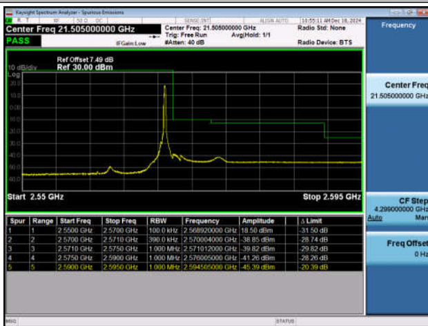
Band7_20MHz_QPSK_21350_1RB#99
