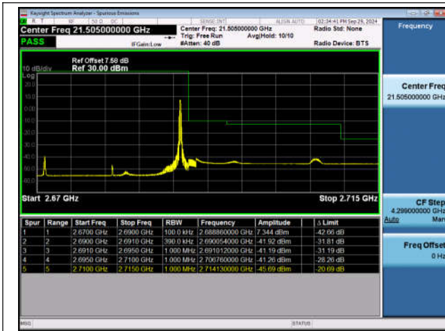
Band41_20MHz_QPSK_41490_1RB#99
