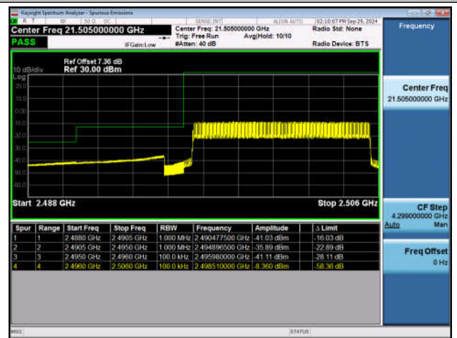
Band41_10MHz_QPSK_39700_50RB#0
