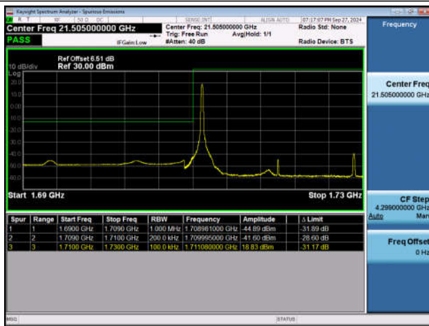
Band66_20MHz_QPSK_132072_1RB#0
