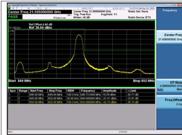
Band5_3MHz_QPSK_20635_1RB#14
