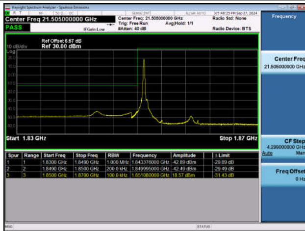
Band2_20MHz_QPSK_18700_1RB#0
