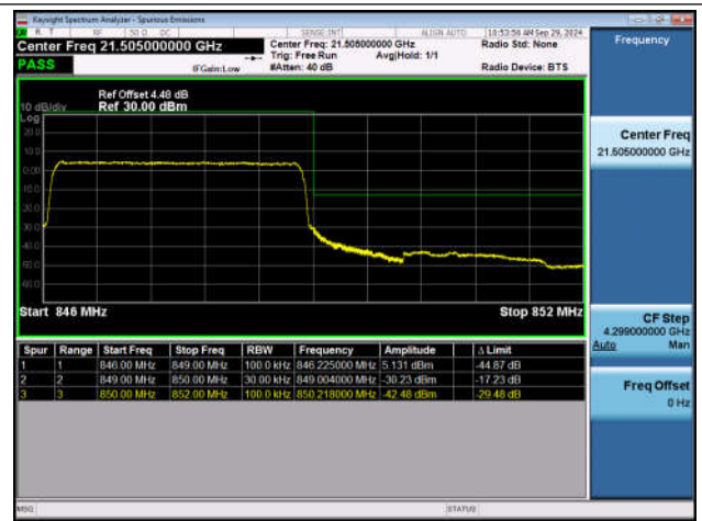
Band5_3MHz_QPSK_20635_15RB#0
