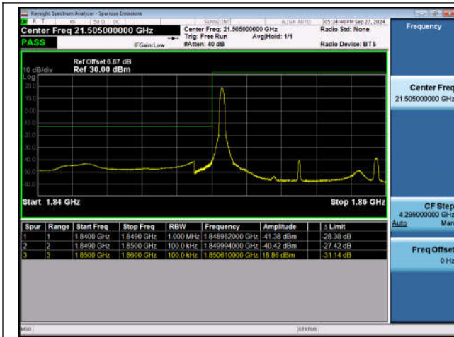
Band2_10MHz_QPSK_18650_1RB#0
