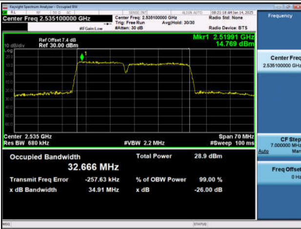
7-7-20MHz-10MHz-QPSK-QPSK-21051-21195-100RB#0-50RB#0-PASS
