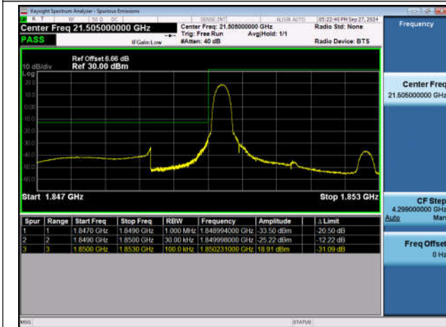
Band2_3MHz_QPSK_18615_1RB#0
