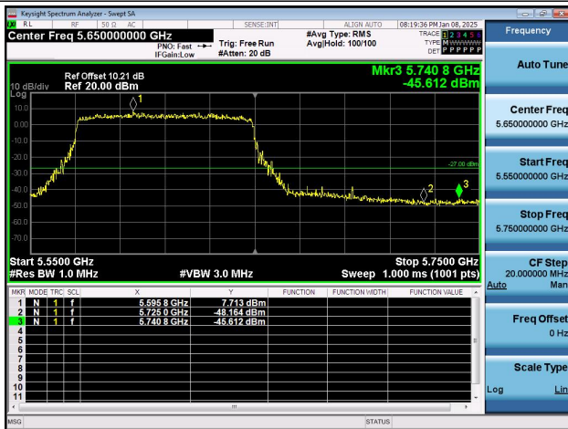
11AX80SISO-Ant1-5610-PASS
