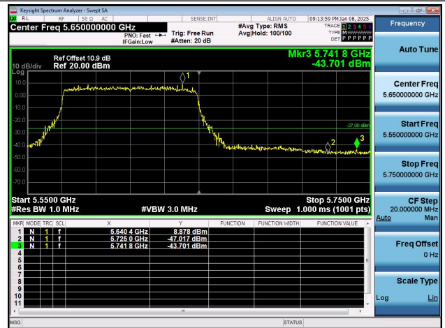
11AX80SISO-Ant2-5610-PASS
