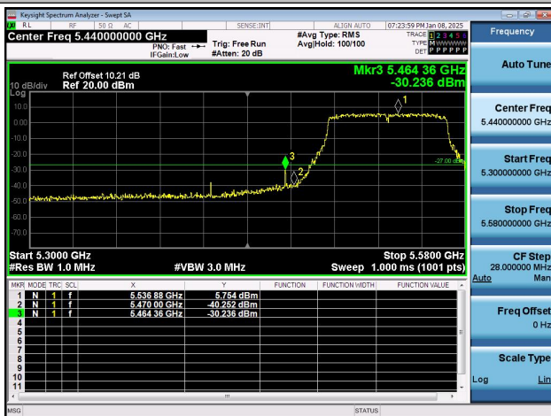
11AC80SISO-Ant1-5530-PASS
