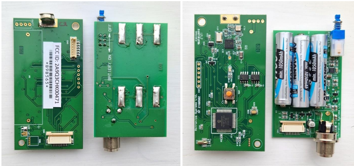
RF Repeater GENII/SRPT/200
