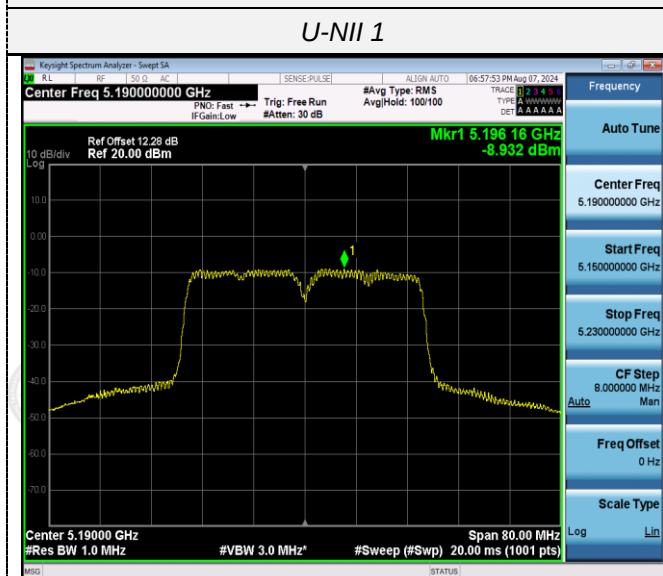
802.11ac(HT40)
