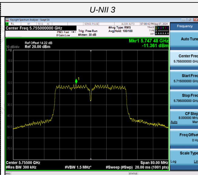
802.11ac(HT40)
