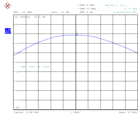
2480 MHz
