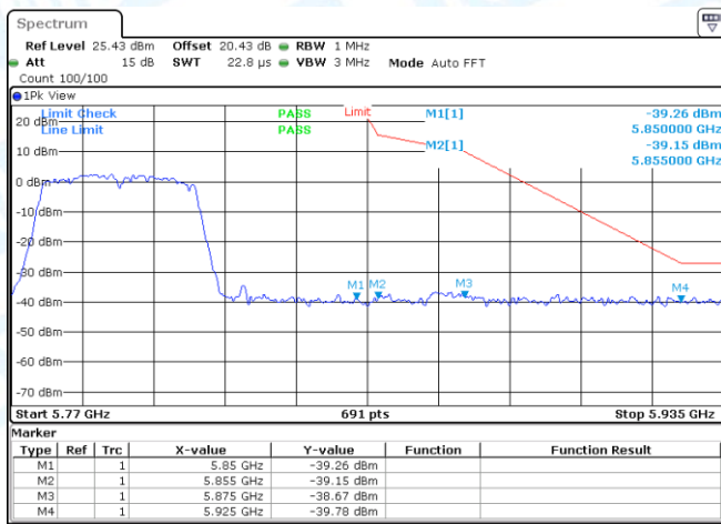
11N40MIMO-Ant1-5755-PASS
