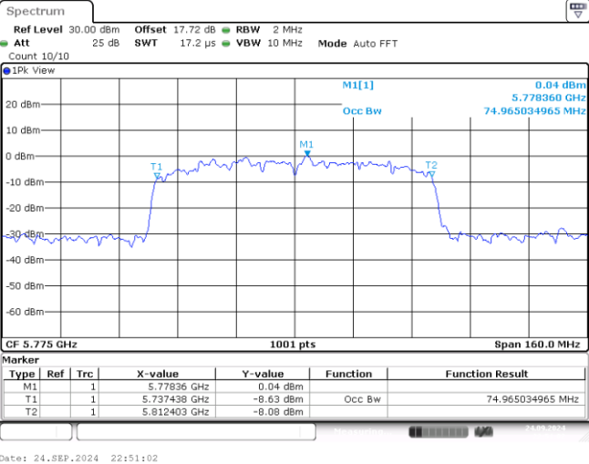
11AC80MIMO-Ant1-5775
