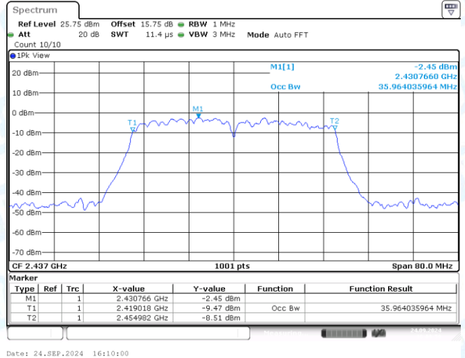
11N40MIMO-Ant2-2437
