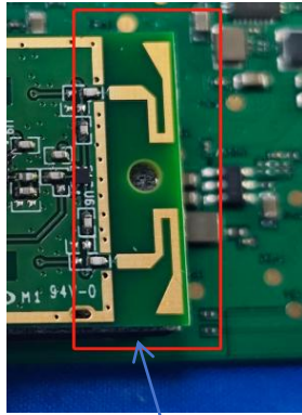
5.8G ant
