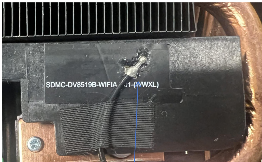
2. 4G&Bluetooth ANT
