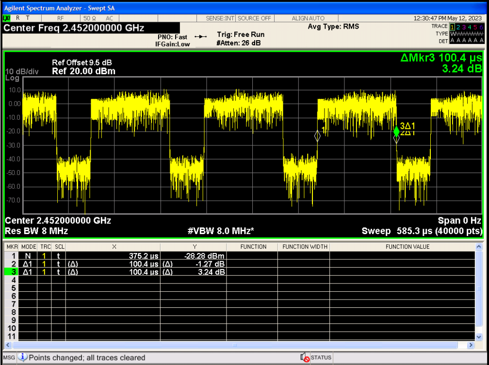
IEEE 802.11n_40MHz_Channel 9
