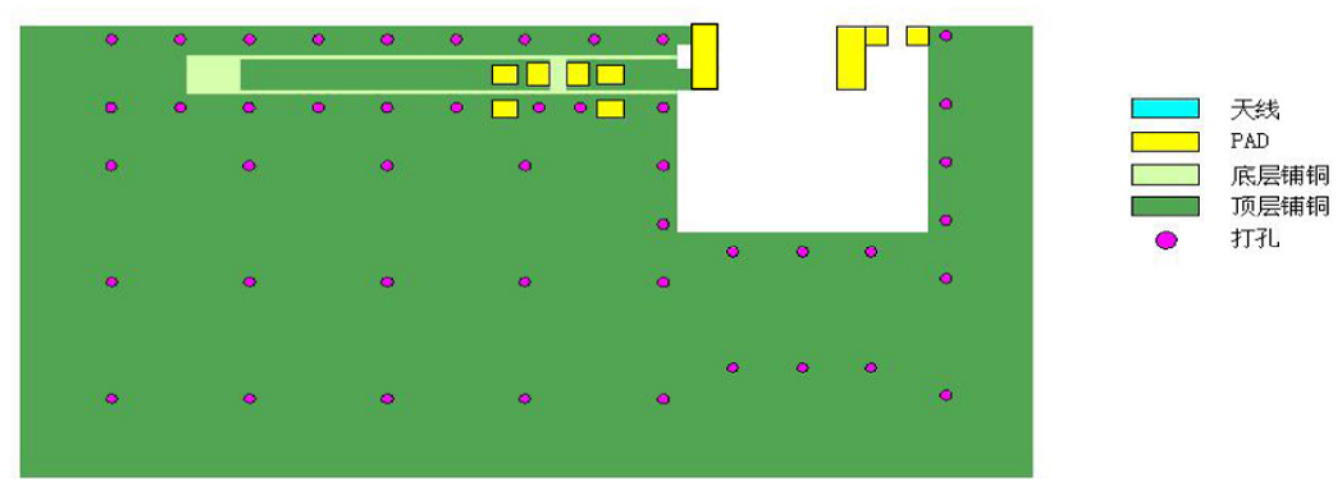
打孔参考示意图
