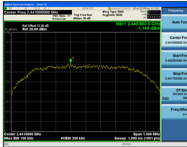
2DH5-Ant1-2441-30~1000--1.15
