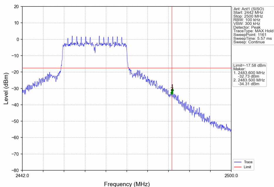
802.11n(HT20) HCH 2462MHz Ant1 (SISO) NTNV
