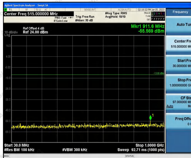
Band25-10MHz-16QAM-26365-1RB#0-Range2:1000~20000MHz
