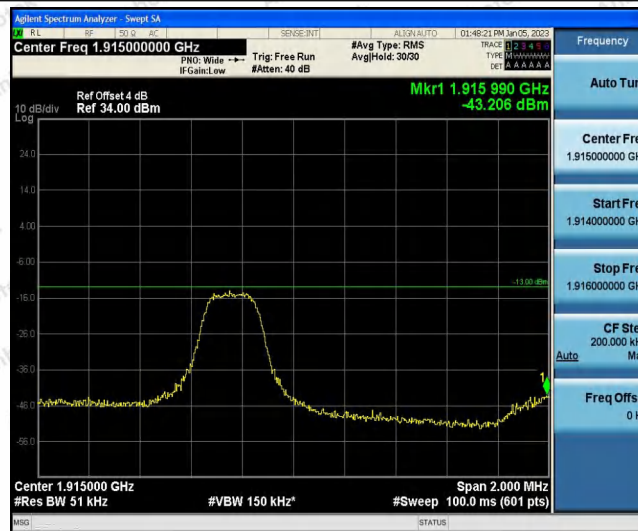
Band25-3MHz-QPSK-26675-1RB#14
