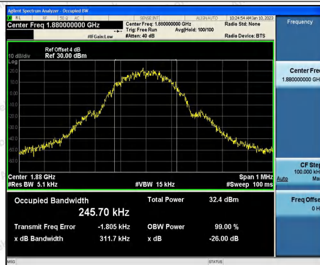
GPRS1900-810
