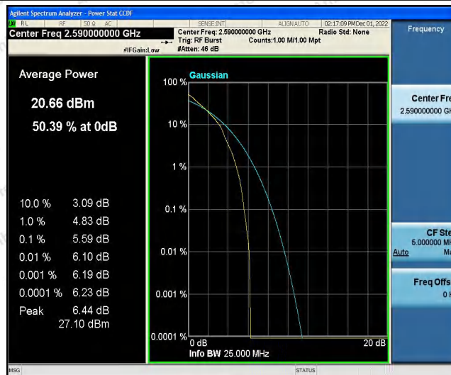
Band41-20MHz-QPSK-40590-100RB#0
