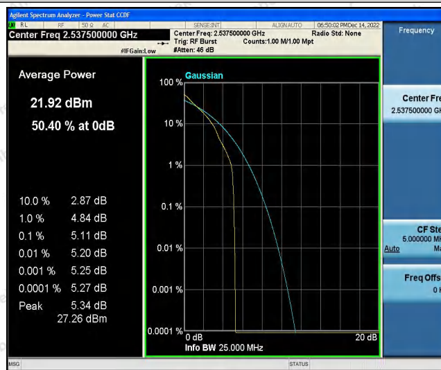
Band41-5MHz-QPSK-40065-25RB#0
