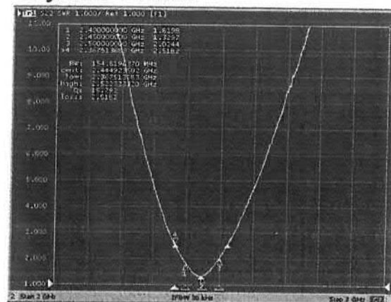
Layout B : VSWR
