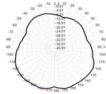
470.0MHz Total(E1-XZ), Max= -0.90dBi
