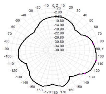
400.0MHz Total(E2-YZ), Max= 0.17dBi
