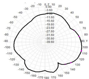
450.0MHz Total(E2-YZ), Max= -0.46dBi
