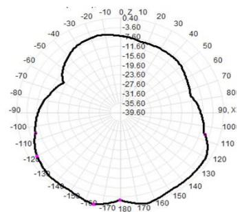
450.0MHz Total(E1-XZ), Max= 0.42dBi
