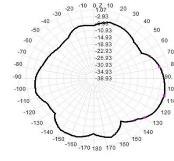
430.0MHz Total(E2-YZ), Max= -0.33dBi
