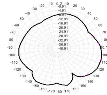
470.0MHz Total(E2-YZ), Max= -1.25dBi
