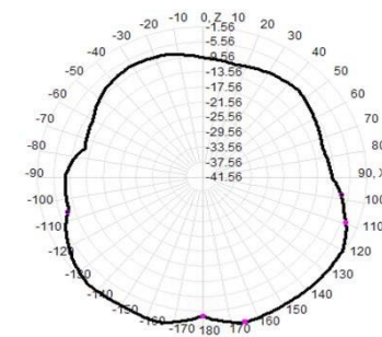
500.0MHz Total(E1-XZ), Max= -1.56dBi
