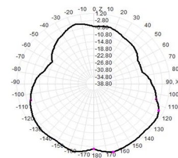
400.0MHz Total(E1-XZ), Max= 1.20dBi
