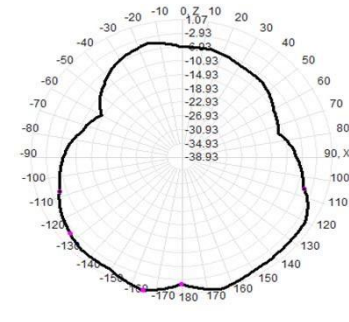
430.0MHz Total(E1-XZ), Max= 1.05dBi
