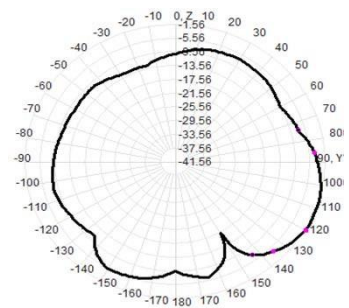
500.0MHz Total(E2-YZ), Max= -1.46dBi
