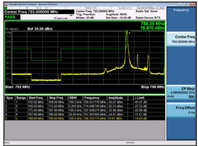
FDD14-5MHz-16QAM-LCH-25RB#0
