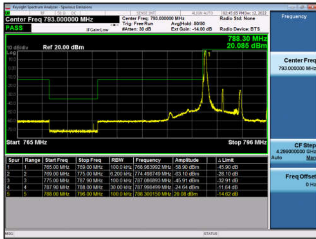
FDD14-5MHz-QPSK-LCH-25RB#0
