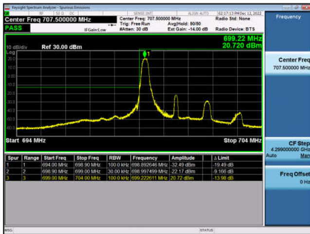
FDD12-3MHz-QPSK-LCH-15RB#0
