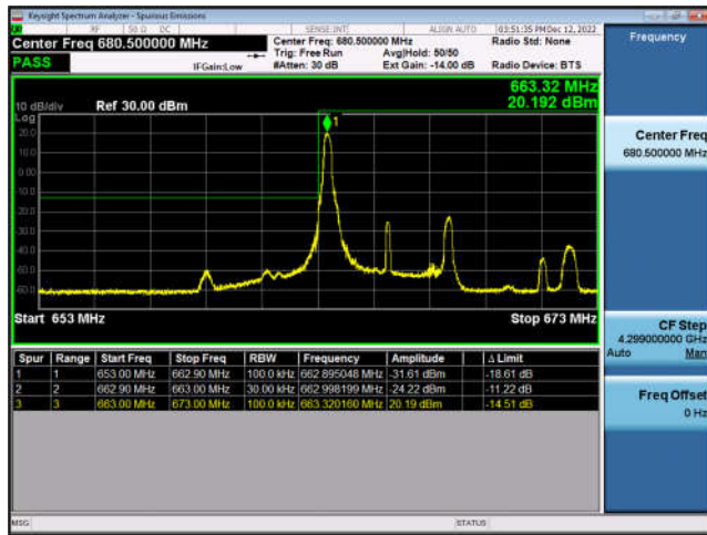
FDD71-5MHz-QPSK-LCH-25RB#0
