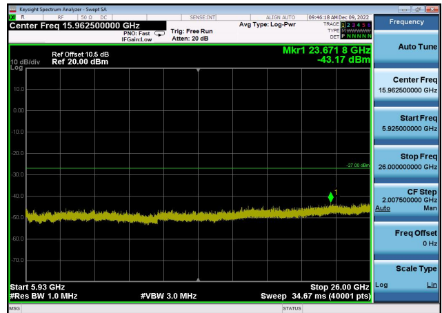
U-NII-3 ,Plot 3,5925MHz~26000MHz-802. 11ac(40MHz),5755MHz,Ant1
