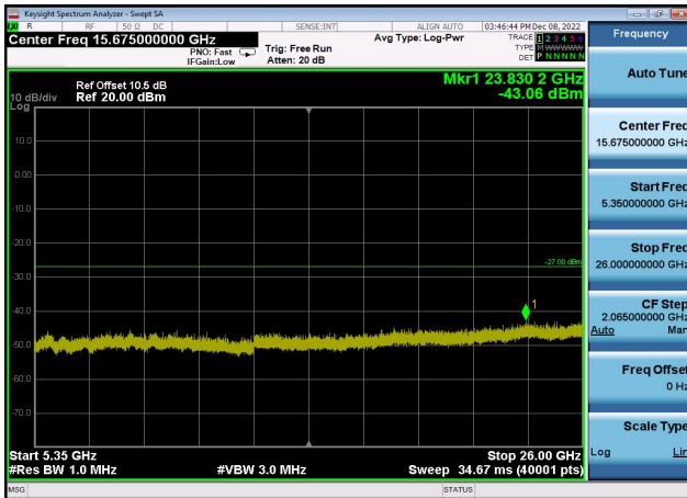
U-NII-1 ,Plot 3,5350MHz~26000MHz-802. 11ac(40MHz),5230MHz,Ant1
