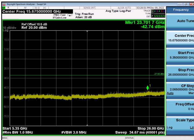
U-NII-1 ,Plot 3,5350MHz~26000MHz-802. 11ac(20MHz),5240MHz,Ant1
