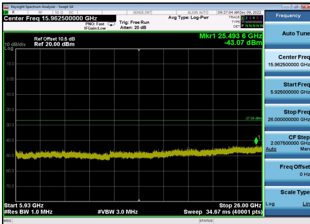
U-NII-3 ,Plot 3,5925MHz~26000MHz-802. 11ac(20MHz),5825MHz,Ant1
