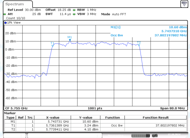
11AX40MIMO-Ant2-5755
